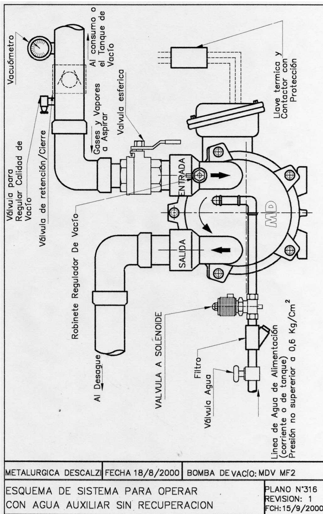
PLANO DE INSTALACIÓN VMF2
